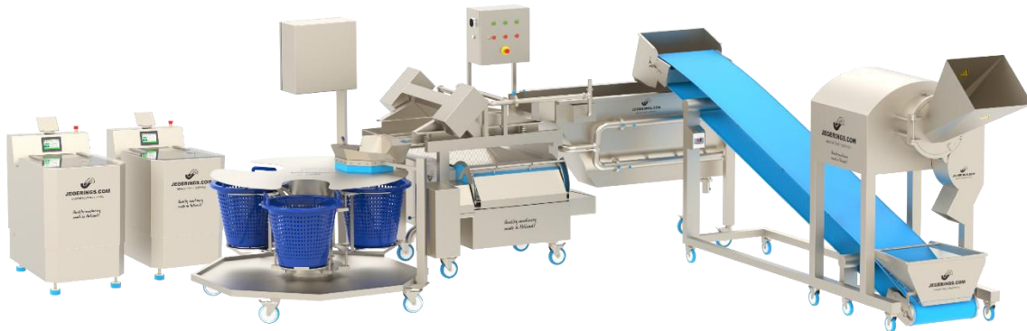
La 3DD en una línea de procesamiento de vegetales para cortar, lavar, (clasificar) y secar vegetales
