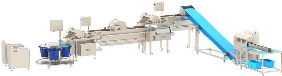
BCM-2450 in einer Gemüseverarbeitungslinie für Schneiden, Waschen und Trocknen von Gemüse
