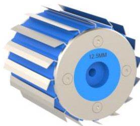
Rouleaux de couteaux hachoirs 12,5 mm
