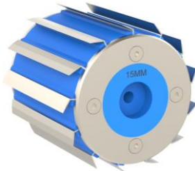
Rouleaux de couteaux hachoirs 15 mm
