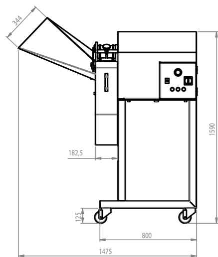
3DD zijaanzicht
